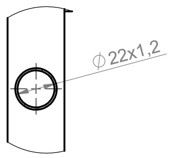
SZCZEGÓŁ C SKALA 1 : 2
